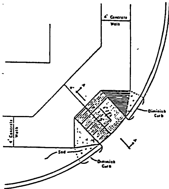
PLAN Scale: 1" = 4'
