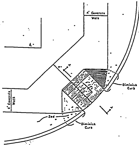
PLAN Scale: 1" = 4'
