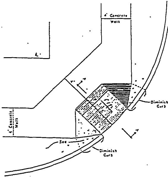
PLAN Scale: 1" = 4'
