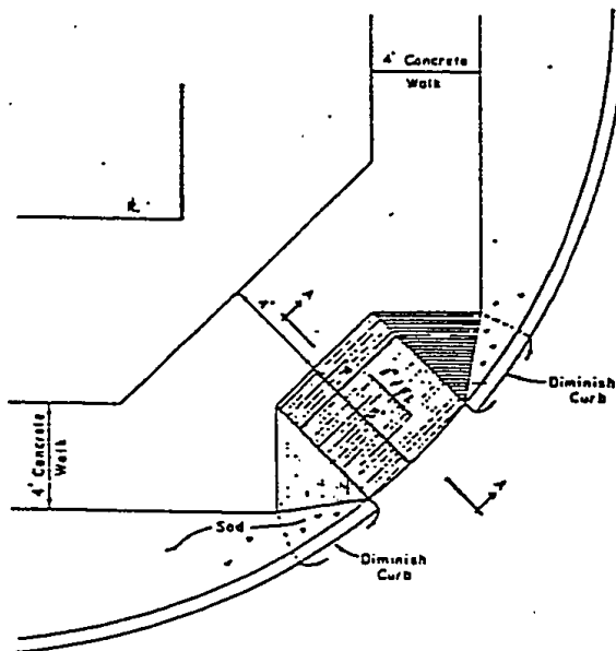
PLAN Scale: 1" = 4'
